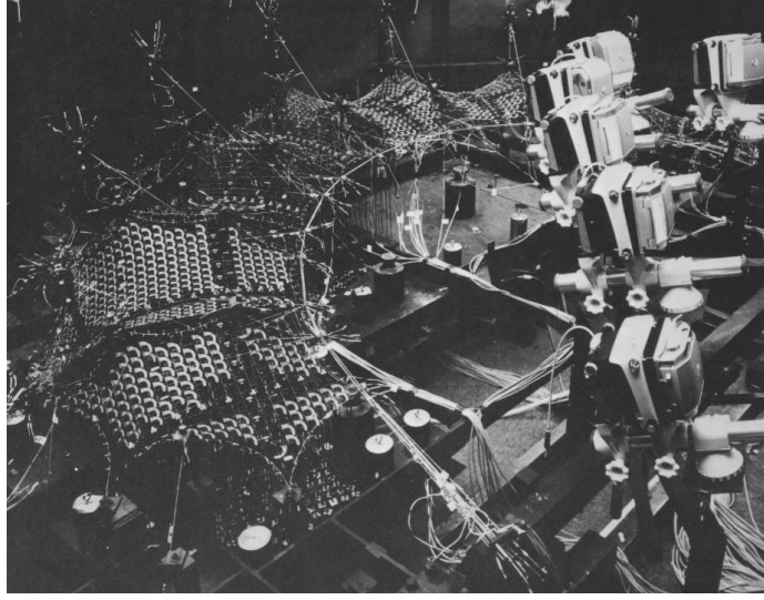
Fotoğraf 5. Frei Otto ve Gunther Behnisch- Münih Stadyumu Fiziksel Modeli
